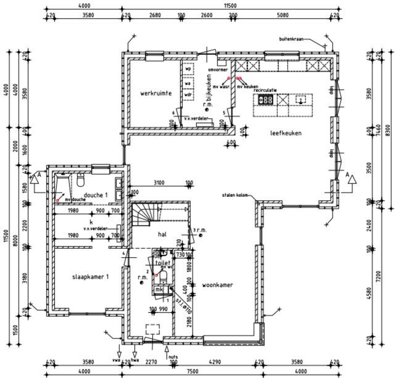
Begane grond
